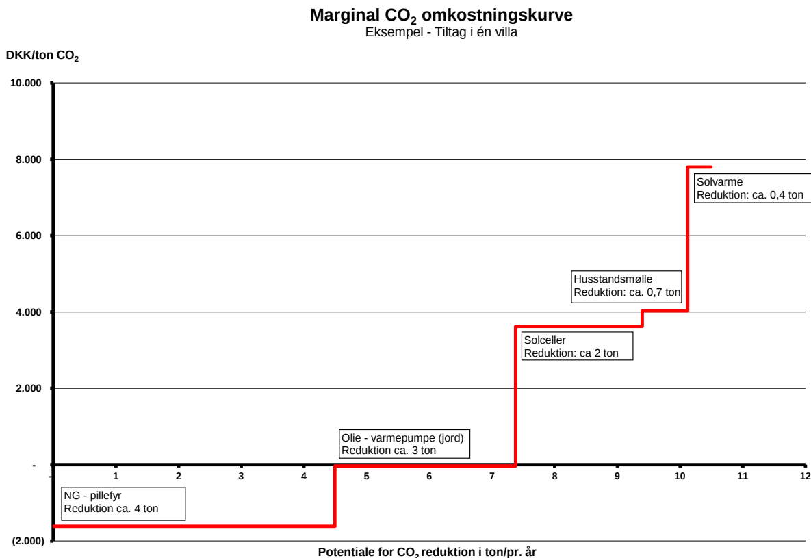
Figur 12: Trappekurve – rangordning af tiltag i en hushold efter kr./reduceret ton CO 2
